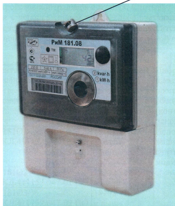
Рисунок 1 - Фотография общего вида и место установки пломбы поверителя счетчиков РиМ 181.08 производства ЗАО «Радио и Микроэлектроника»
